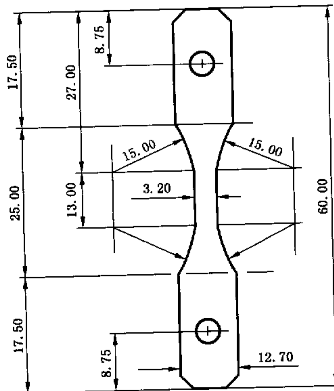
图 C.1 L型试样的尺寸图
