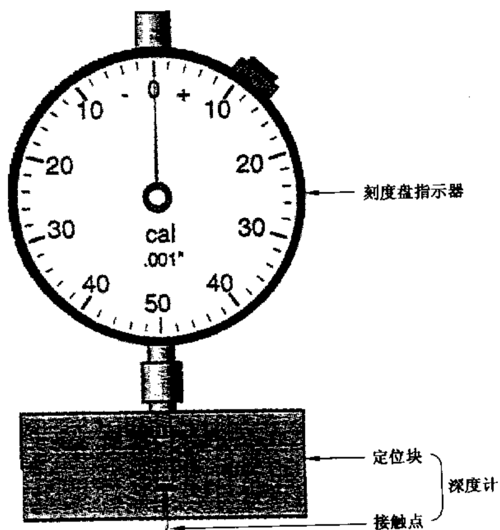
图 F.1 粗糙度高度试验装置结构图
