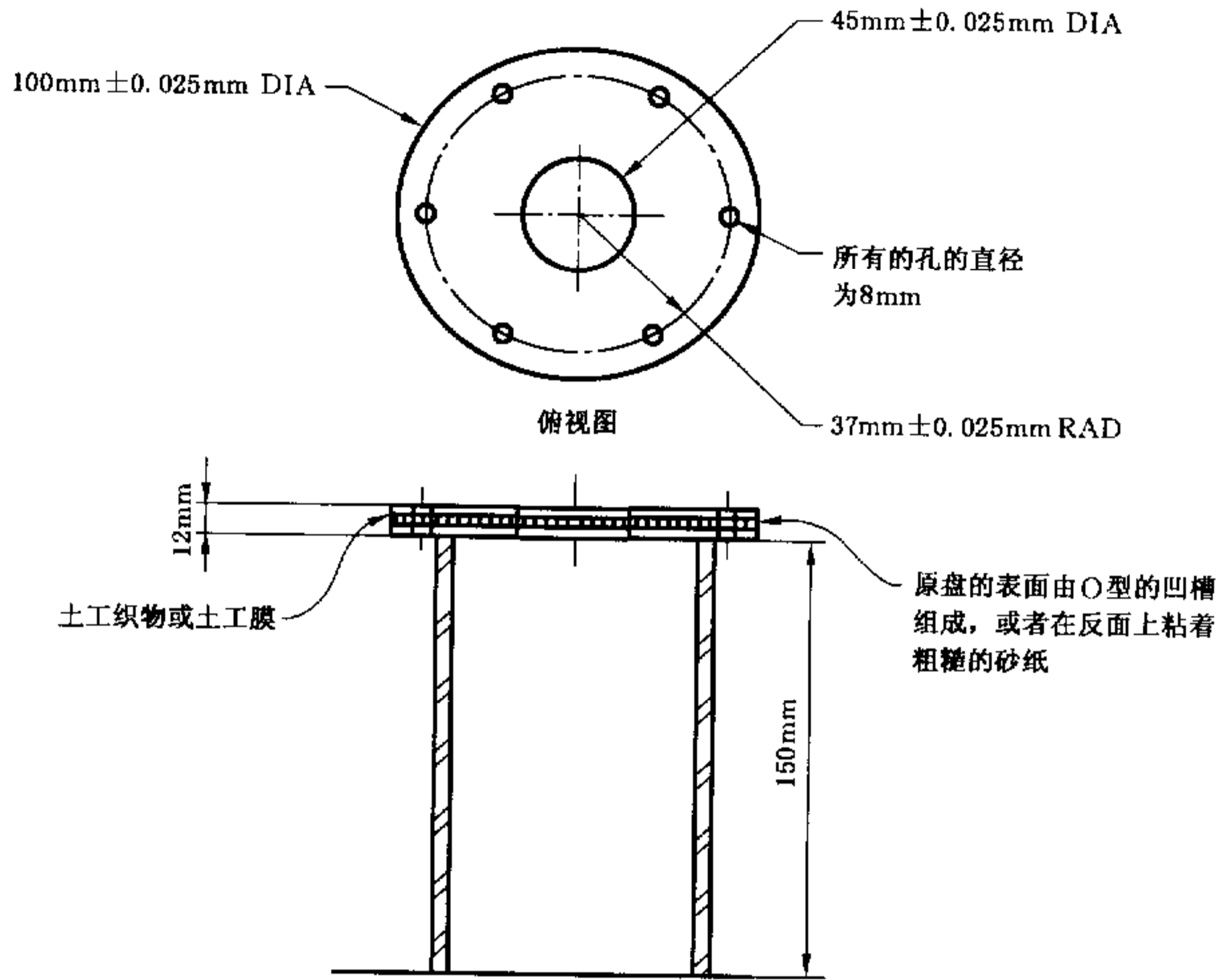
图 B.2 试验安装细节(未按比例)
