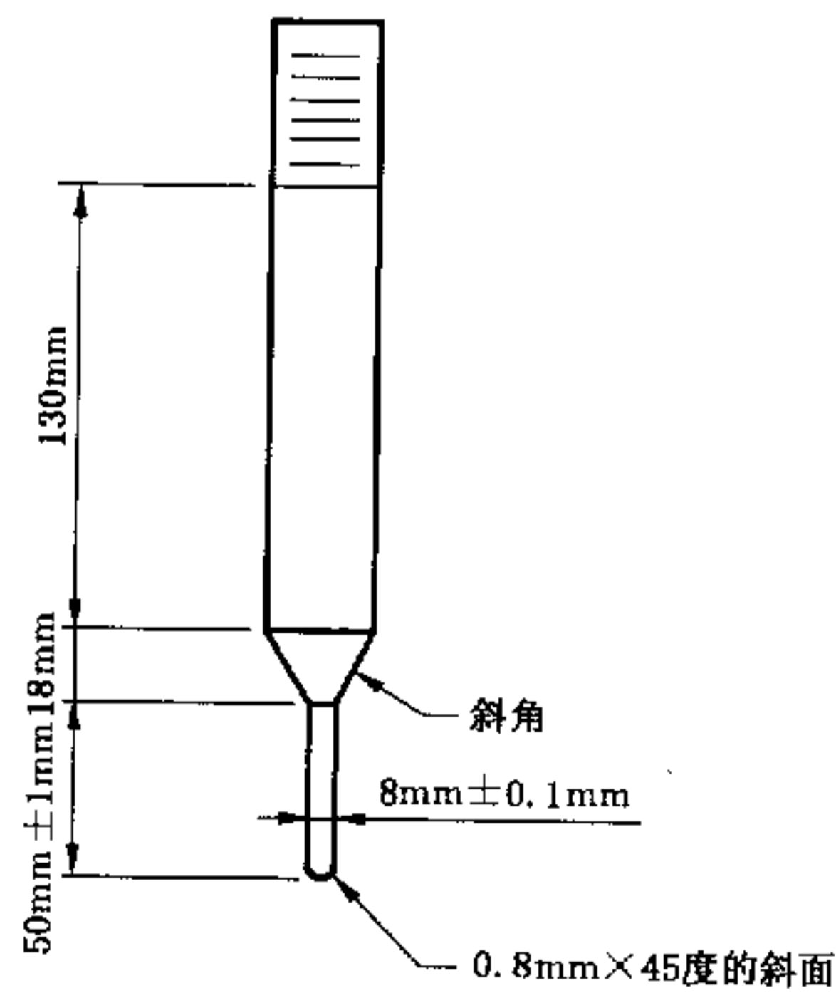
图 B.3 试验穿刺针细节(未按比例)
