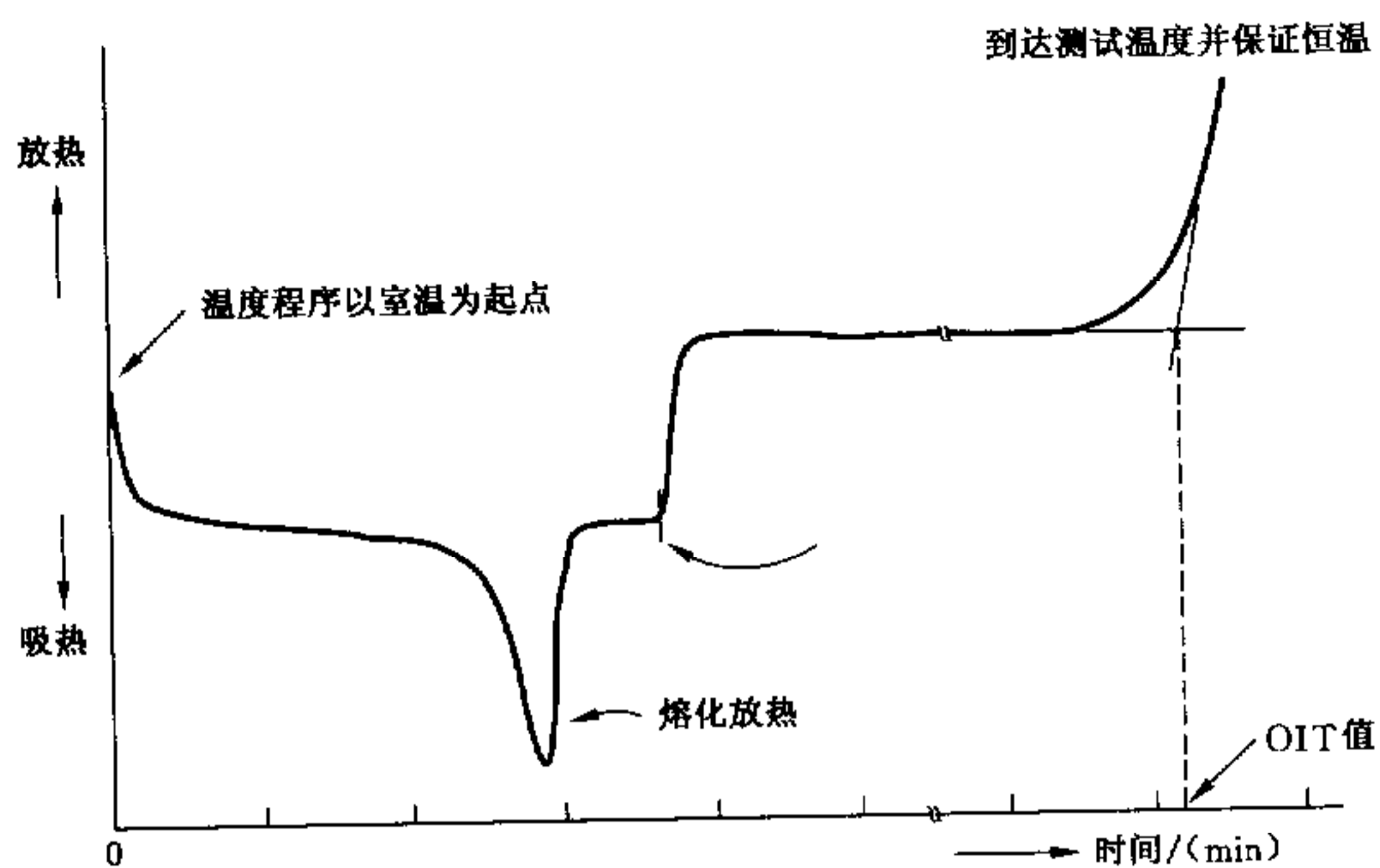
图 E.1 试验温度曲线图
