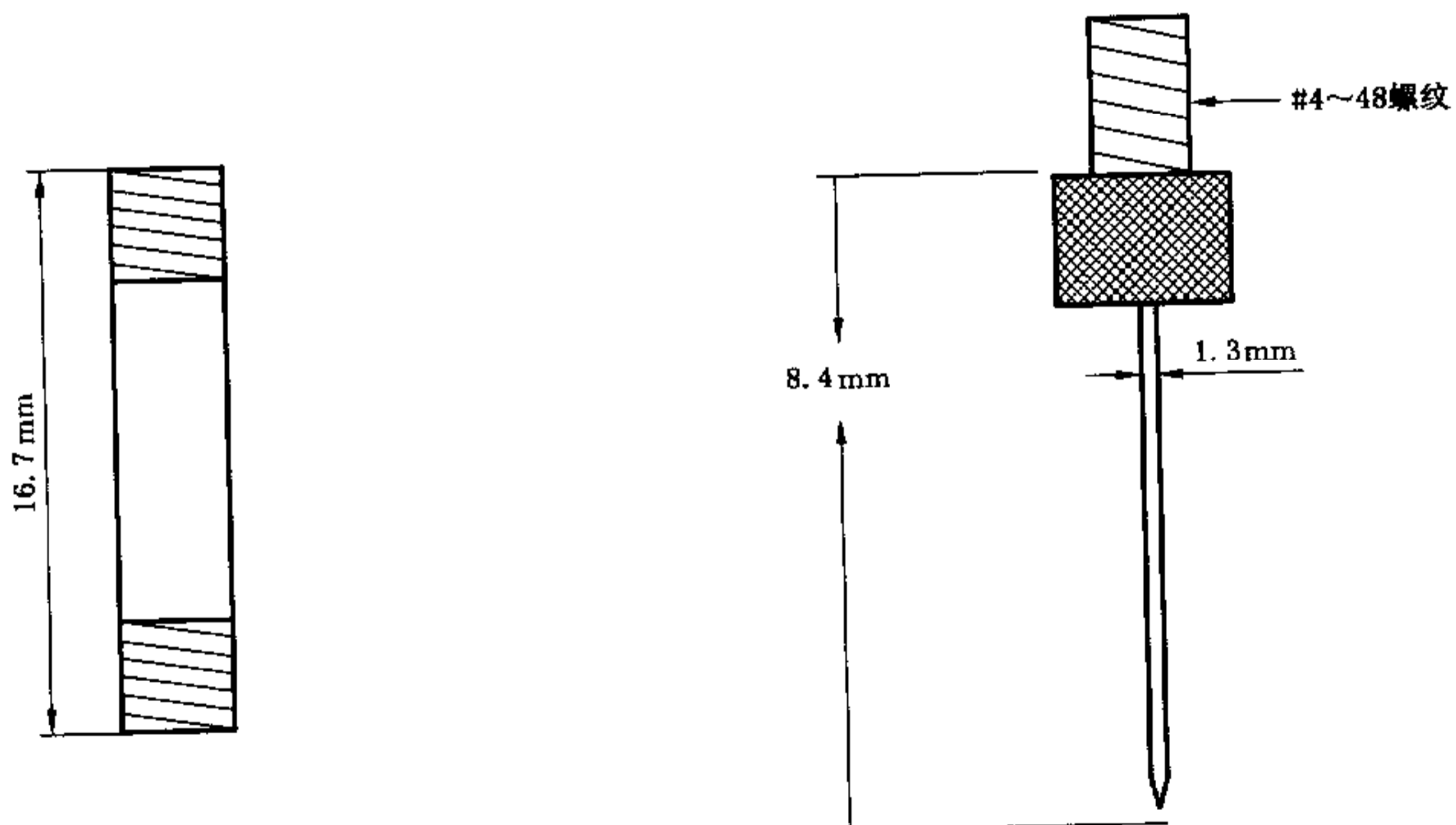
图 F.3 接触点尺寸
