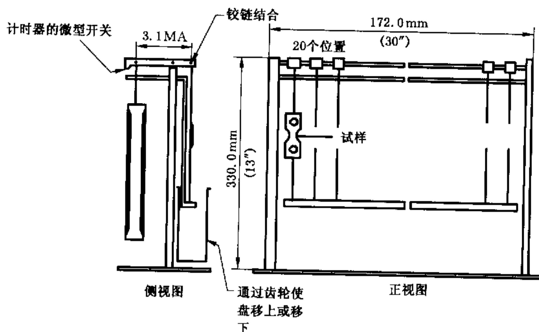
图 C.2 有 20 个试样测试位置的恒载施加装置
