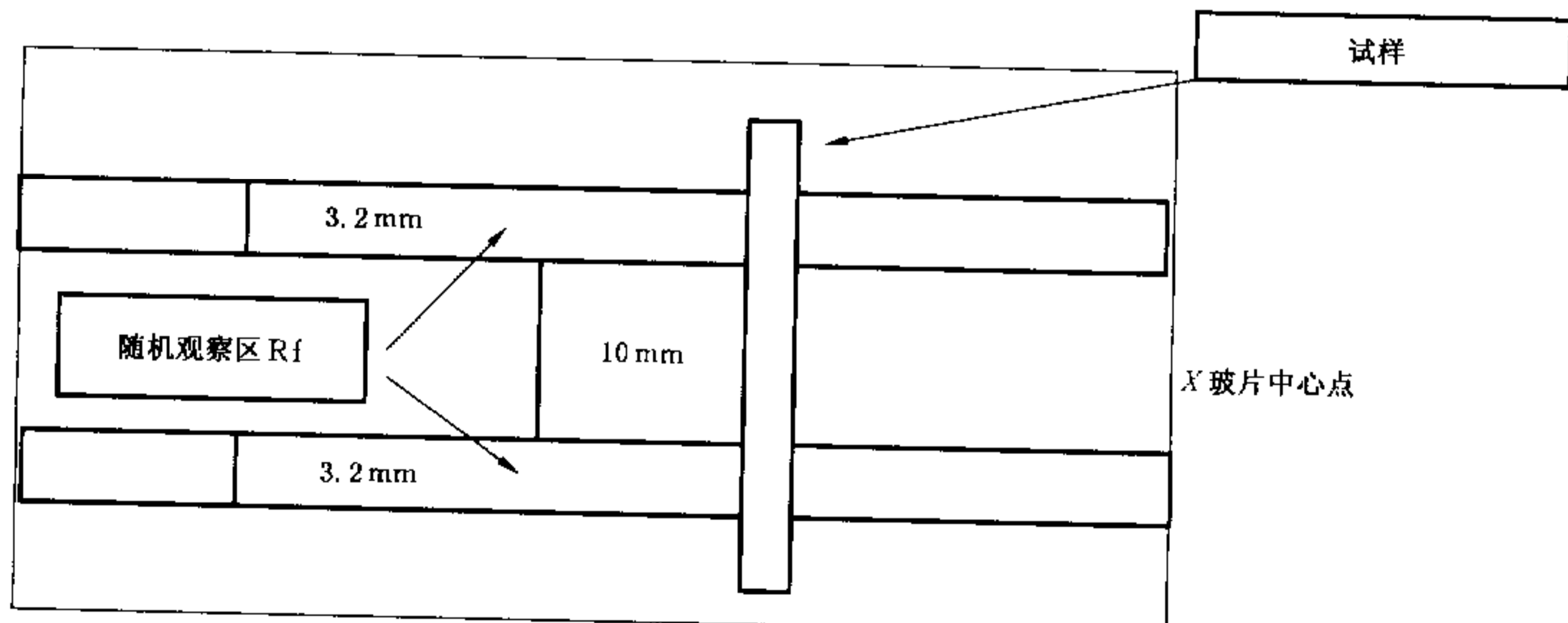
图 D.1 显微镜盖玻片轮廓图
